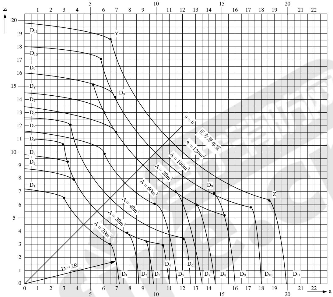
图 E 探测器安装间距的极限曲线
