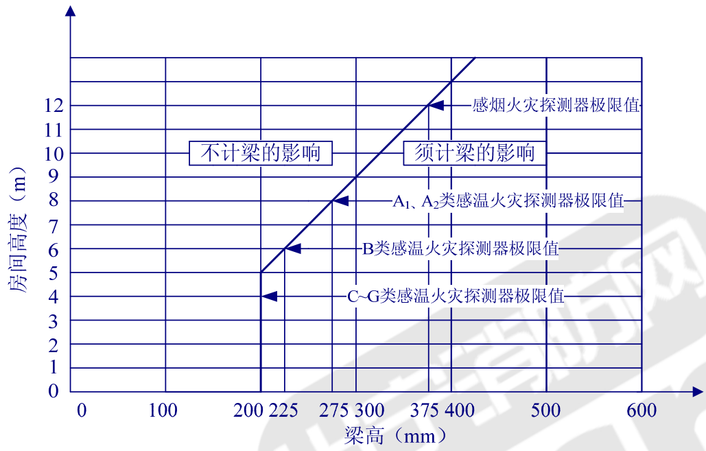
图 F 不同高度的房间梁对探测器设置的影响
